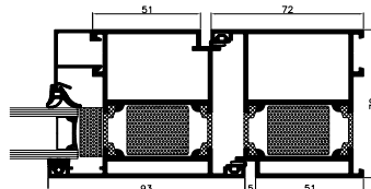
przekrój przez drzwi MB-70 HI
